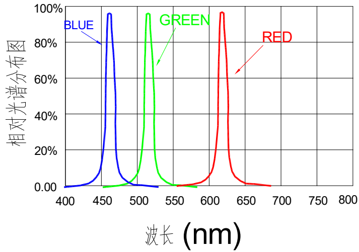
波长特性
